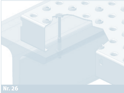
Direktverschraubung Nr. 26
